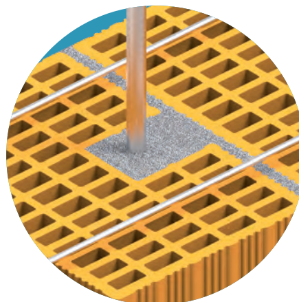
particolare
