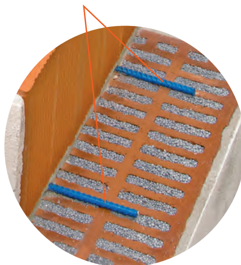
Armatura orizzontale
