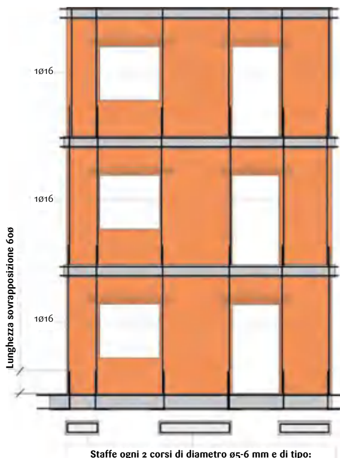
Staffe ogni 2 corsi di diametro \phi 5-6 \text{ mm} e di tipo:
